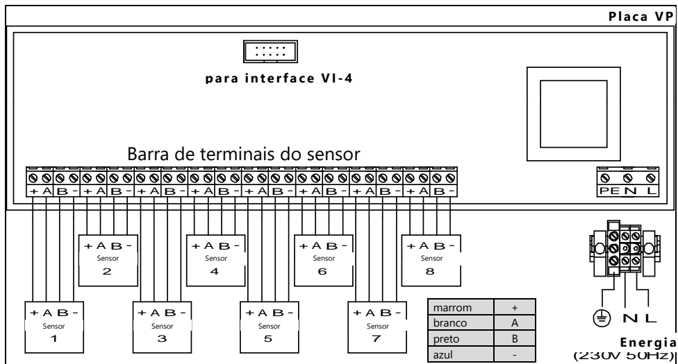
Figura 1: VISY-Command 8 com placa VP-1 para 8 sensores
