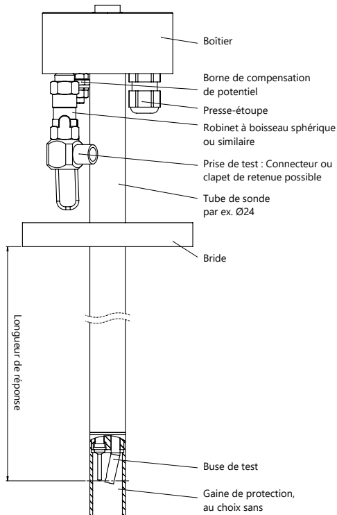
Image 1.4g : LS 300 FSP
