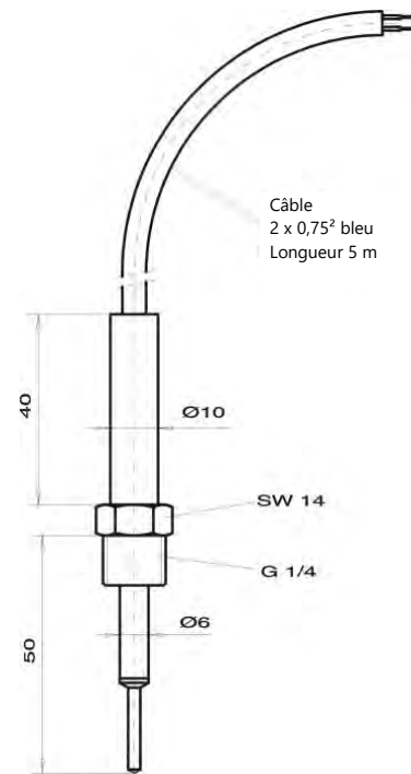
Image 1.4j : LS 300 EB6
