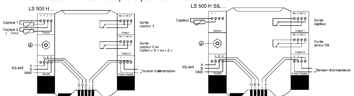
Image 5b : Transducteur de mesure dans boîtier enfichable sur rail
