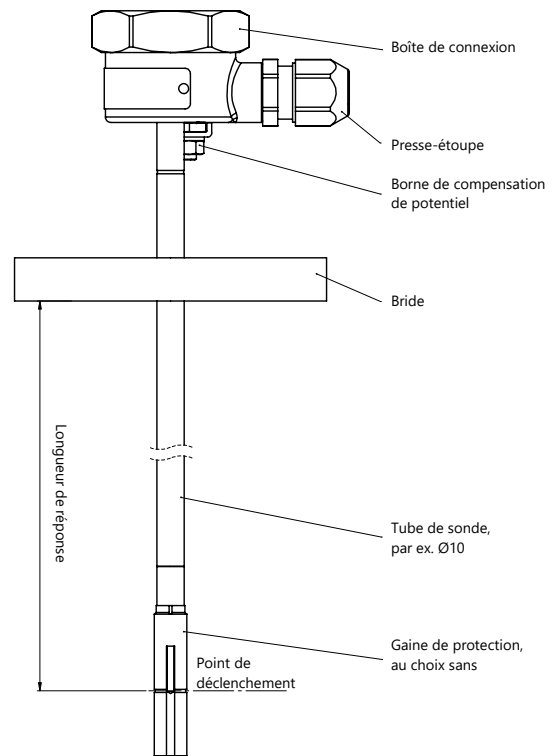
Image 1.4b : LS 300 F
