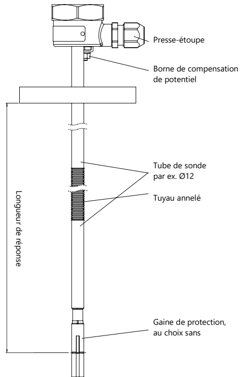
Image 1.4i : LS 300 FX
