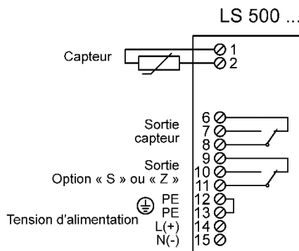
Image 5a : Transducteur de mesure dans boîtier de montage mural
