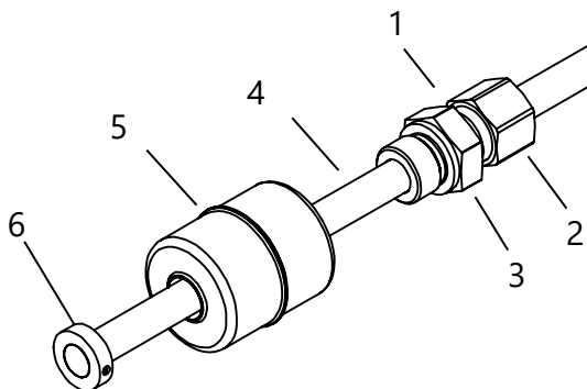
Abbildung 3: Montage mit Einschraubkörper
